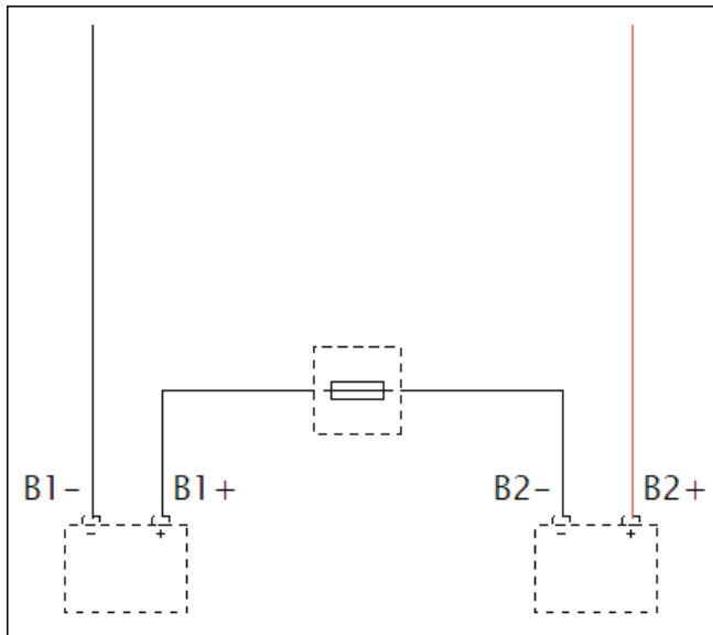
Seriekoppling, batterier: 24 V
