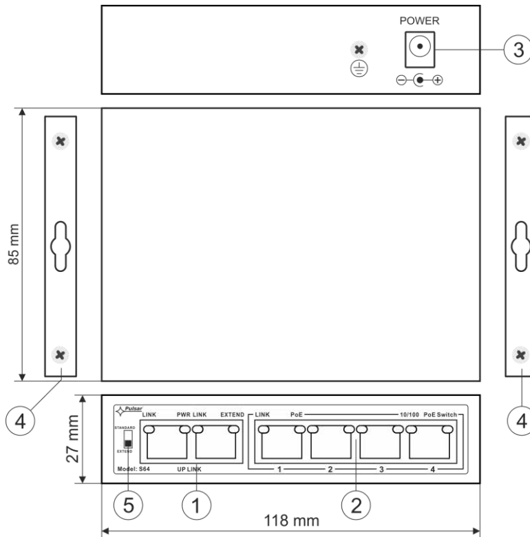
Bild. 3. Switchen.
