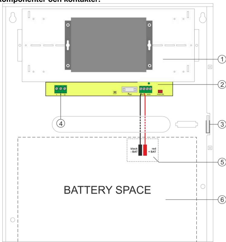
Bild 2. Höljet.
