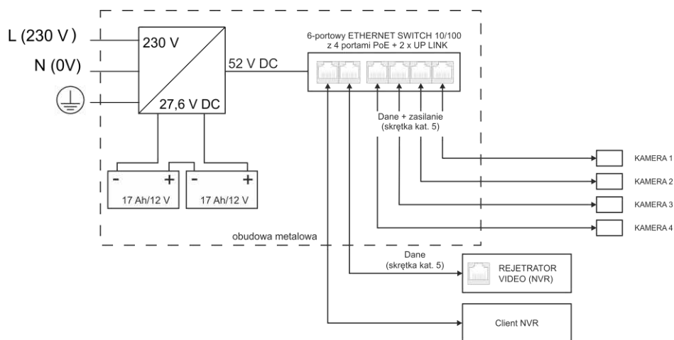
Bild 1. Blockschema.
