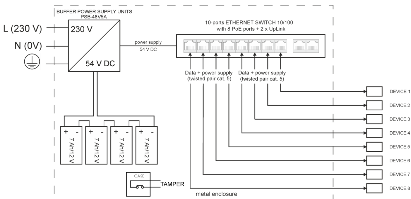
Bild 1. Blockschema.
