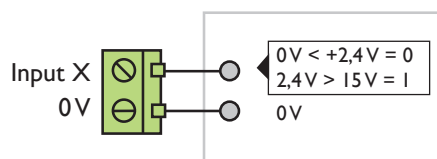
Fig. 3: Digitala ingångar
