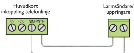
Fig. 1: Telefonuppkoppling
