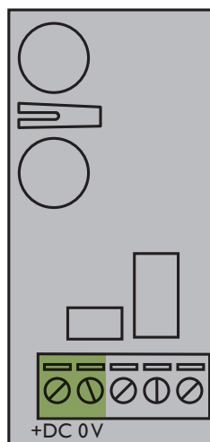
Fig. 11: Strömförsörjning på laddkortet
