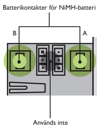
Fig. 13: Batterikontakter
